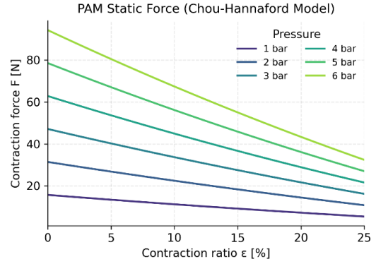
그림 2. Chou-Hannaford 모델 기반 PAM 정역학
